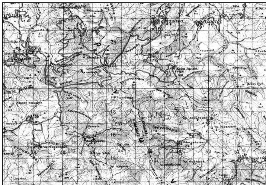
Αποσπασμα χάρτου 1:100.000 περιοχής Αγίου Βασιλείου Πάρωνας
